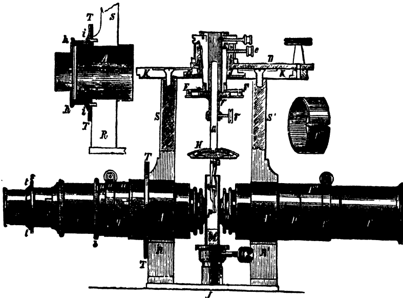
412H.
